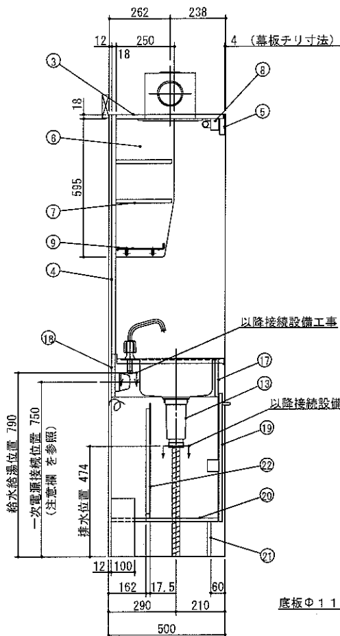
(フロントカバー取付後の寸法 502)
