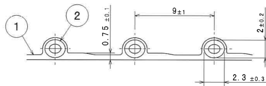
A部詳細 スケール：4/1
